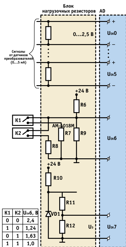
Рис. 6. Схема блока нагрузочных резисторов
