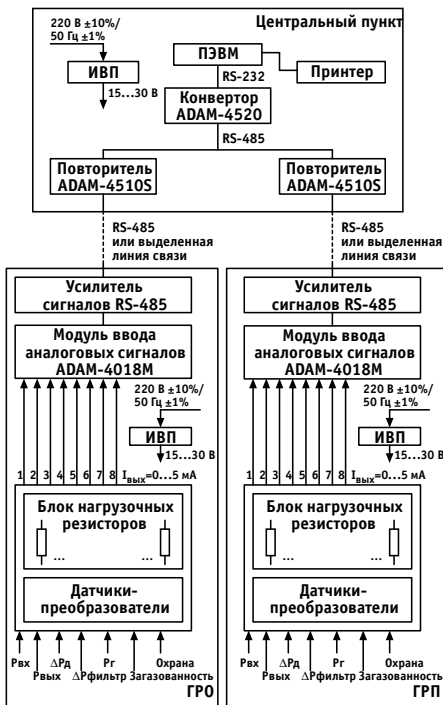
Рис. 2. Структура АИС-ГАЗ
